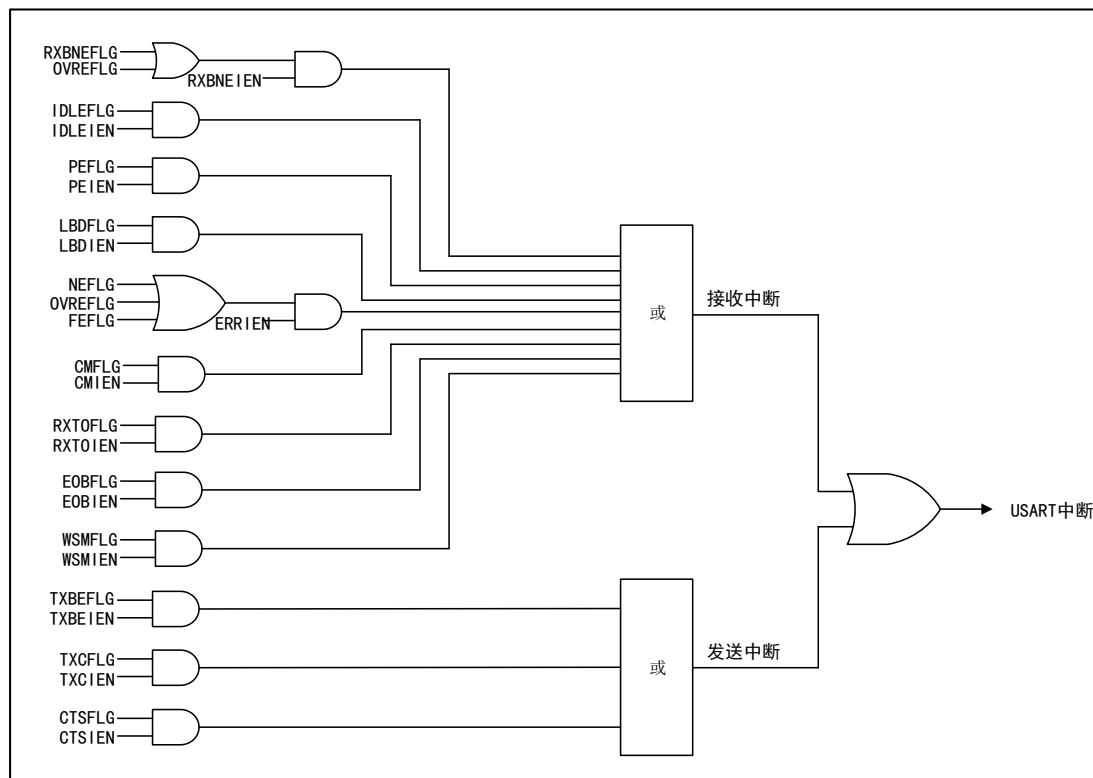
图 102 USART 中断映射
