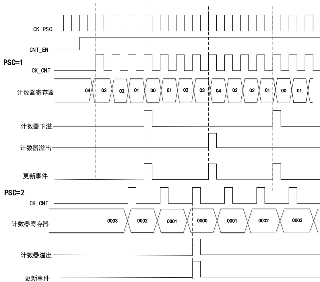
图 28 中央对齐模式下，分频因子为 1 或 2 的时序图
