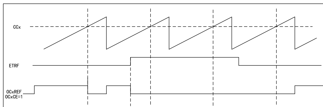
图 87 OCxREF 时序图
