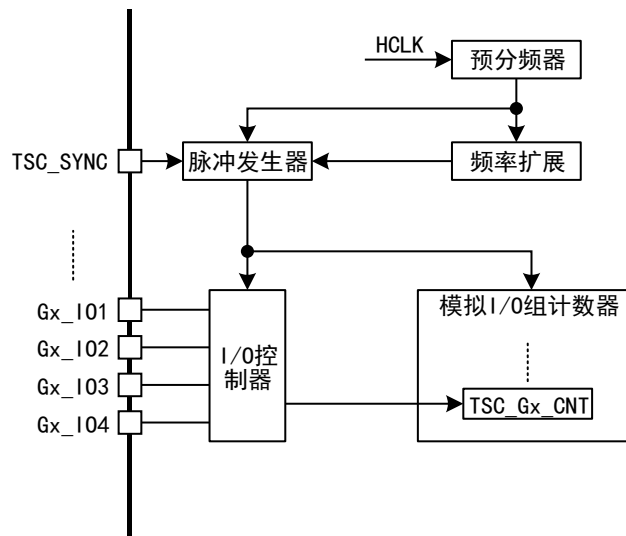
图 129 结构框图
