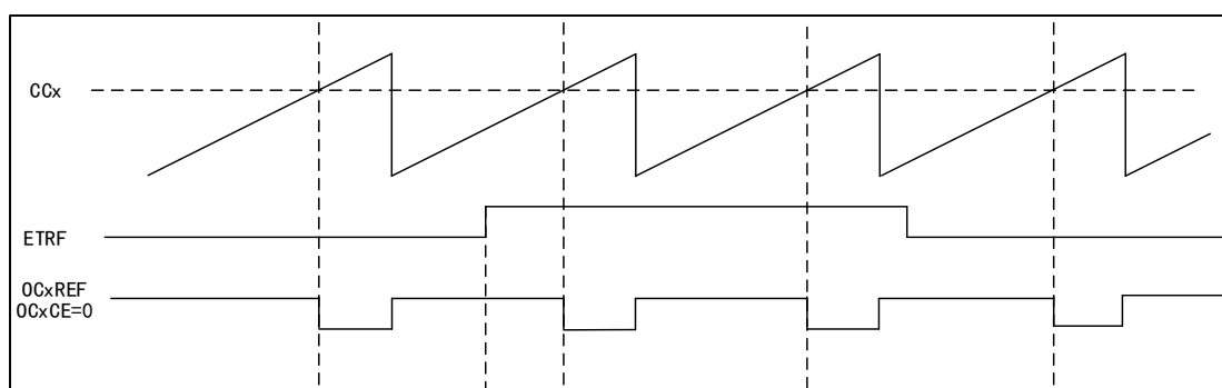
图 86 OCxREF 时序图
