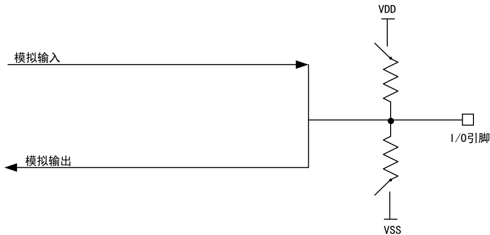
图 21 模拟功能 I/O 结构
