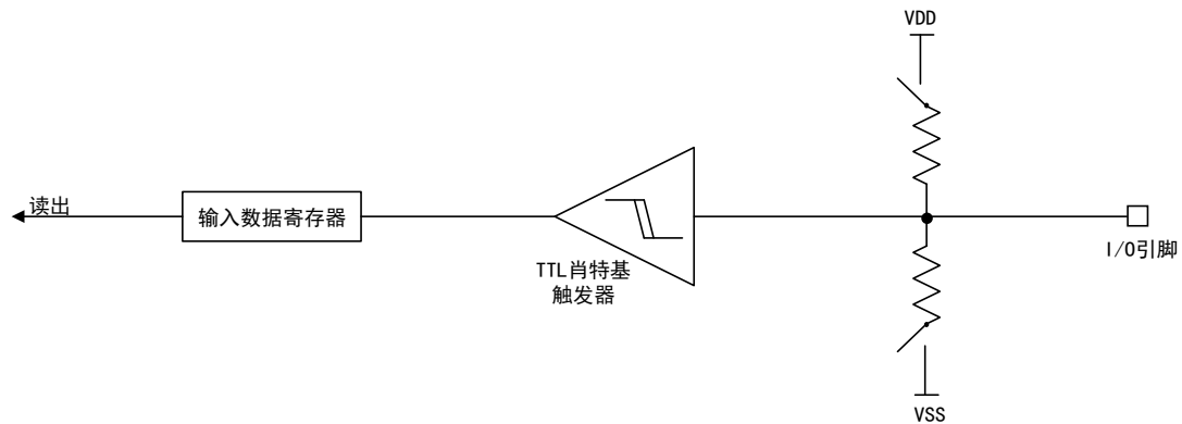
图 18 输入模式 I/O 结构
