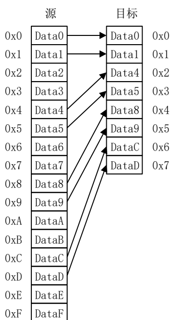
图 15 源为 32bits 目标为 16bits 的传输宽度
