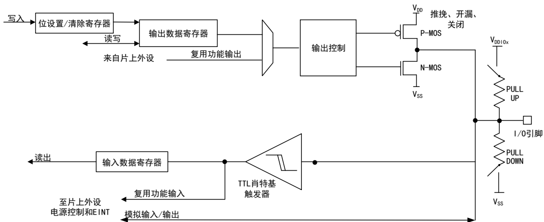
图 17 GPIO 结构框图
