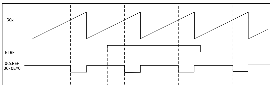
图 39 OCxREF 时序图
