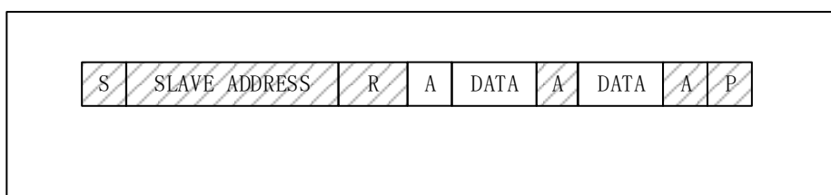
图 107 主机由从机读取数据
