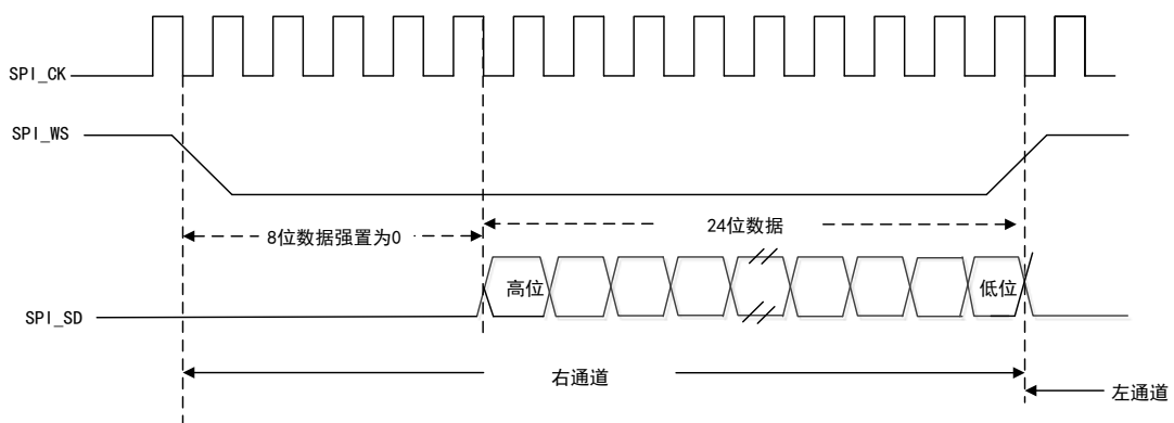
图 120 LSB 对齐标准波形（24 位数据）
