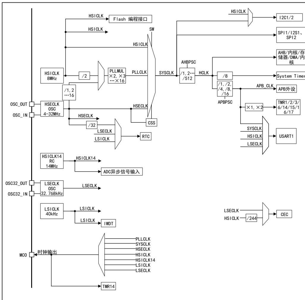
图 4APM32F051x6x8 时钟树
