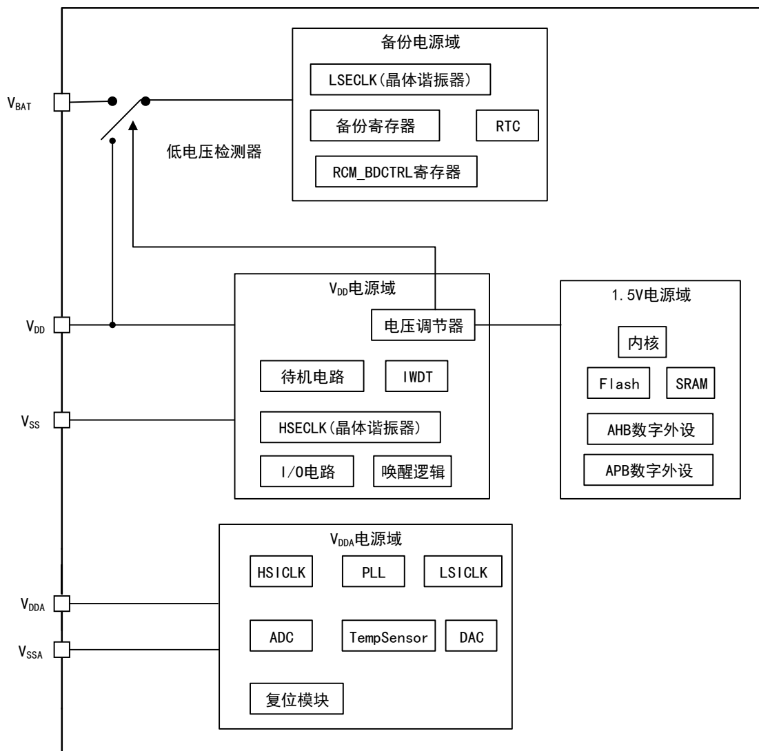
图 6 电源控制结构框图
