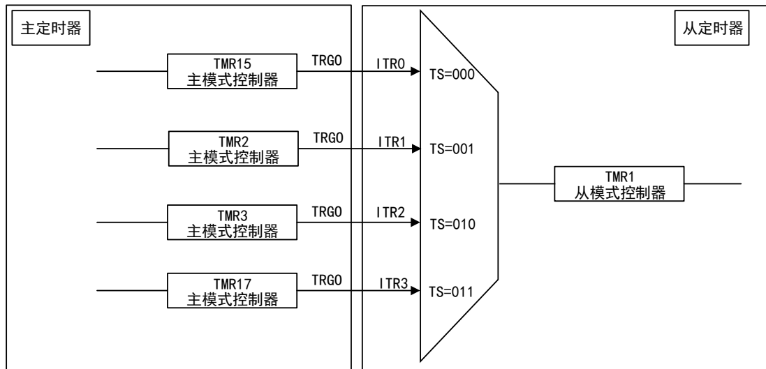
图 85 定时器 1 主/从模式的例子
